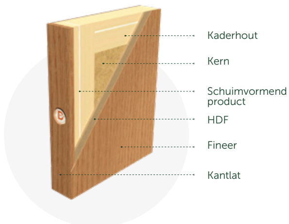
Type B Overplakte kantlat met fineer
