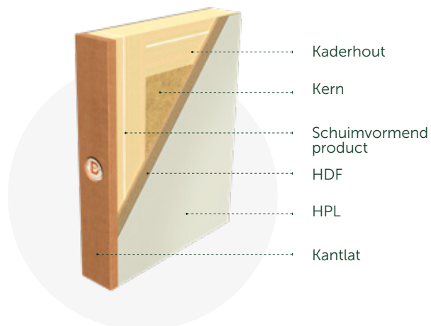
Type C Zichtbare kantlat met HPL
