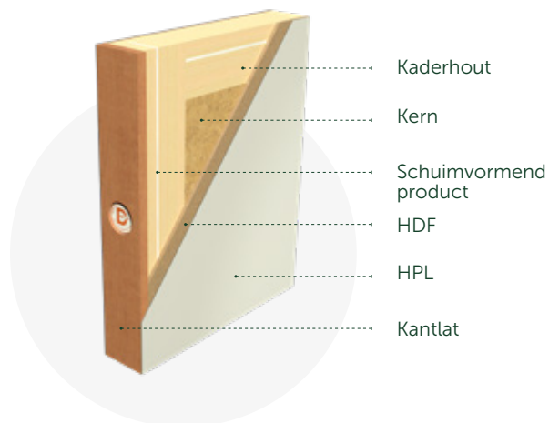
Type B Overplakte kantlat met HPL
