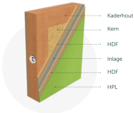
Deur met inlage (lood, aluminium, staal)
