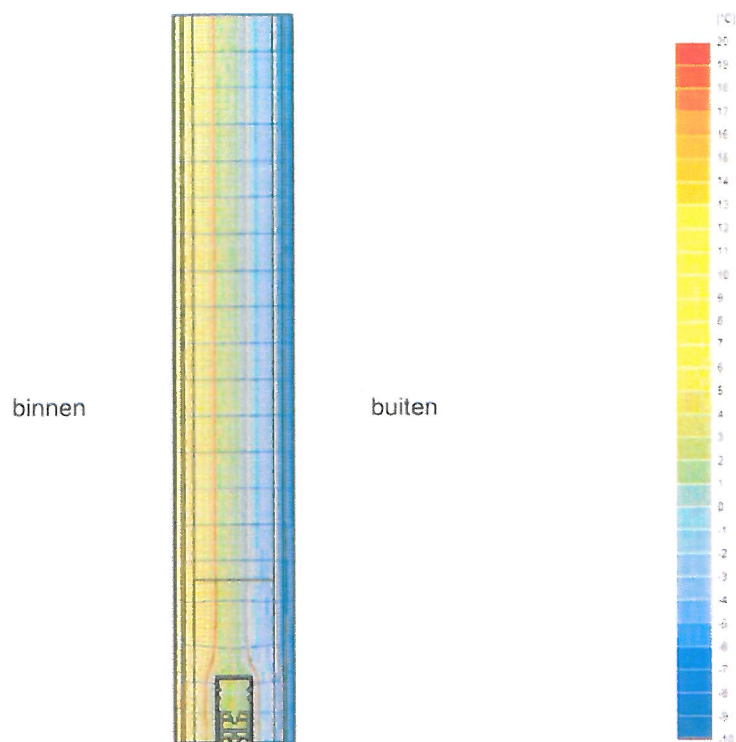
Figuur 4 Grafische weergave warmtedoorgang doorheen zone 4 (binnentemperatuur = 20 °C, buitentemperatuur = -10 °C)
